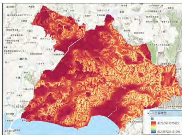
日射量解析
