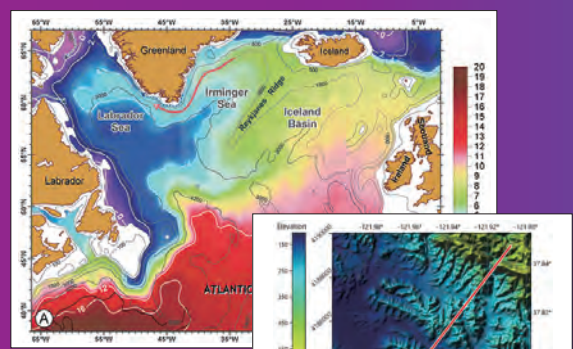
▲海洋温度分布
