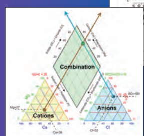
▶パイパーの概念図(トライリニア)
